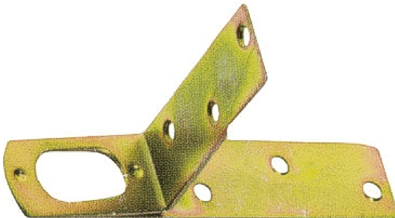
ASOLE A SQUADRA X PENSILI A.Z. 76
