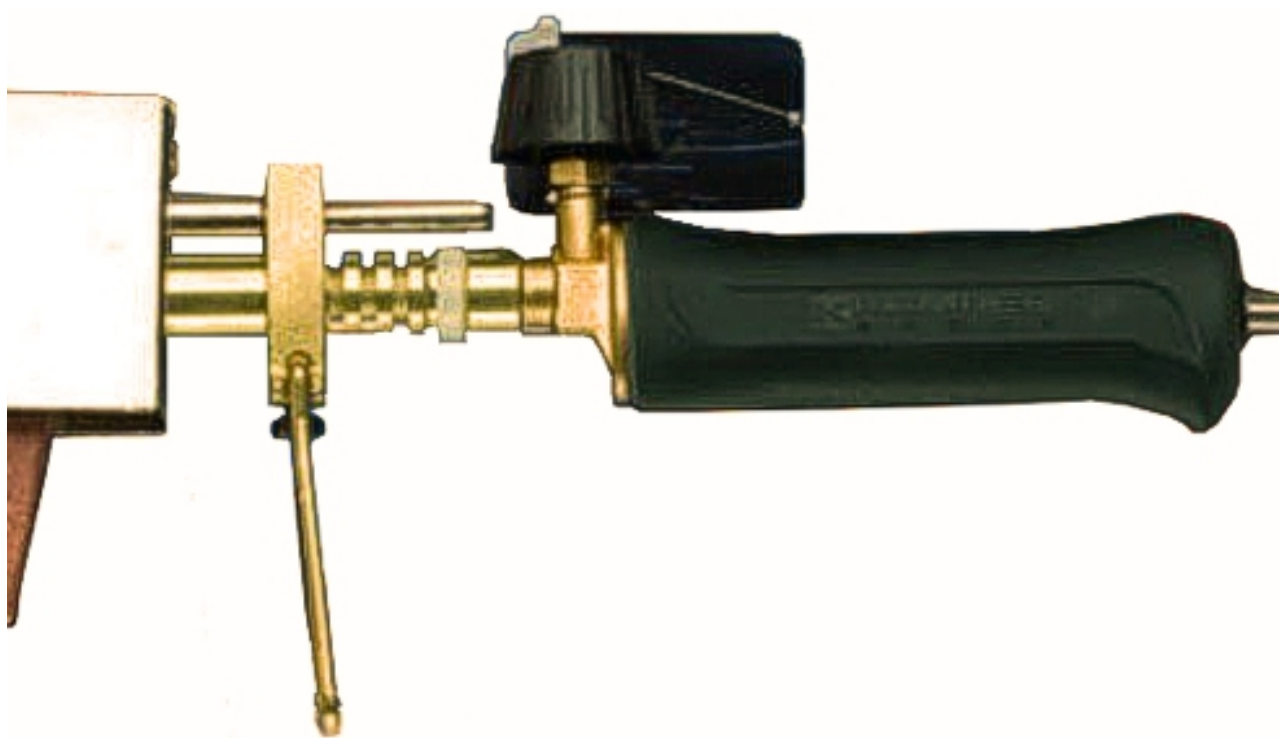
CANNELLI GAS C/MAZZA RAME BRUCIATORE MM.22 1217R
