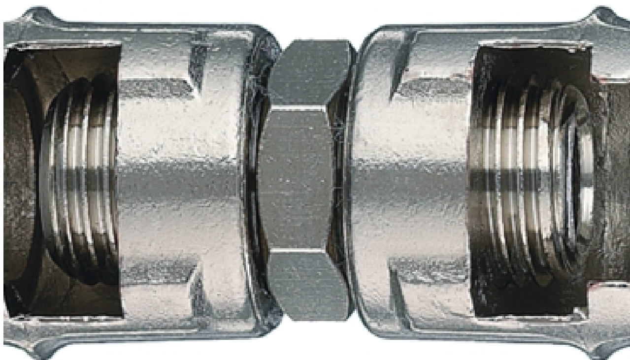
RACCORDI ARIA DI GIUNZIONE C/DADI C. 12A AH011101
